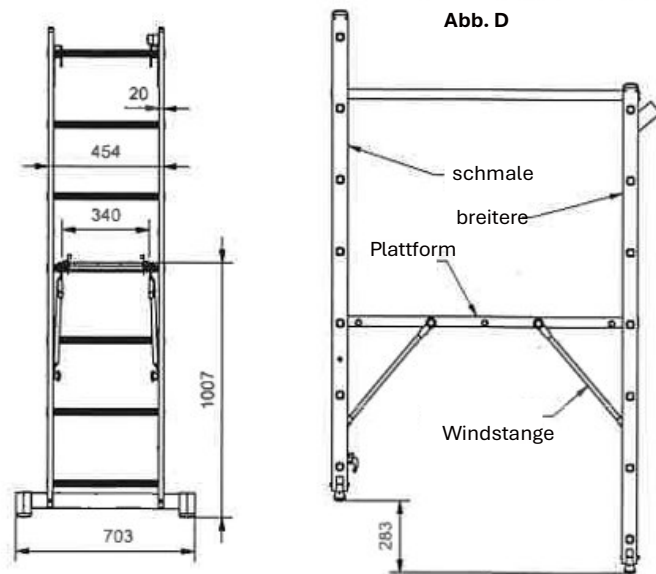
2) Arbeitsplattform für Arbeiten auf Treppen
